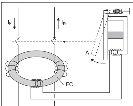
Рис. 2. Упрощенная схема УЗО: FC — ферромагнитный кольцевой сердечник дифференциального трансформатора тока; A — толкатель расцепителя контактной системы
